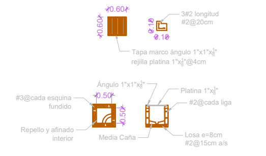
Detalle caja aguas lluvias
