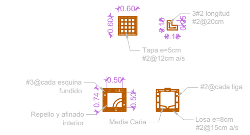
Detalle caja agua residual
